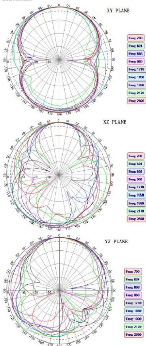
LTE Antenna
