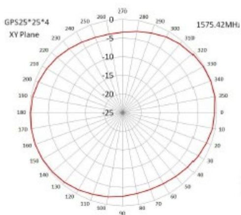
GPS Antenna
